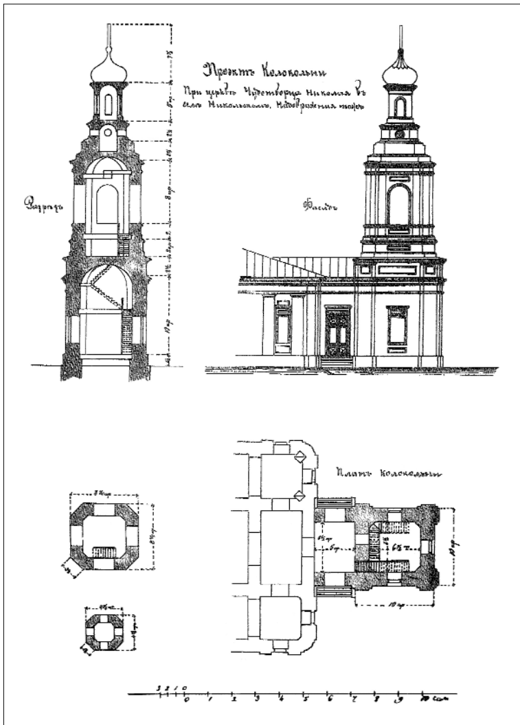
Проект колокольни церкви в селе Надовражино. 1884 год. Из фондов ЦИАМ.
