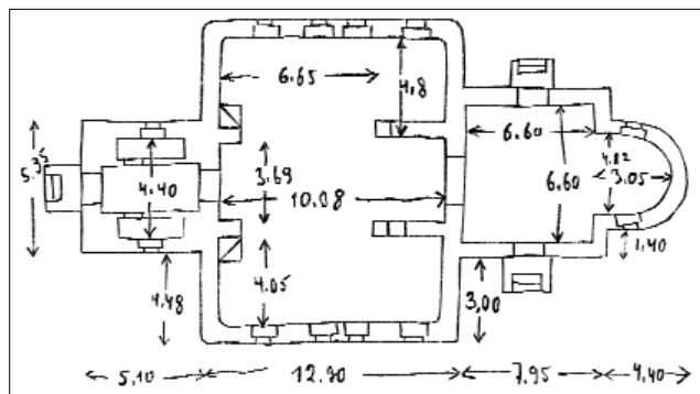
План каменной Крестовоздвиженской церкви. 1933 год. Из фондов ЦГАМО.
