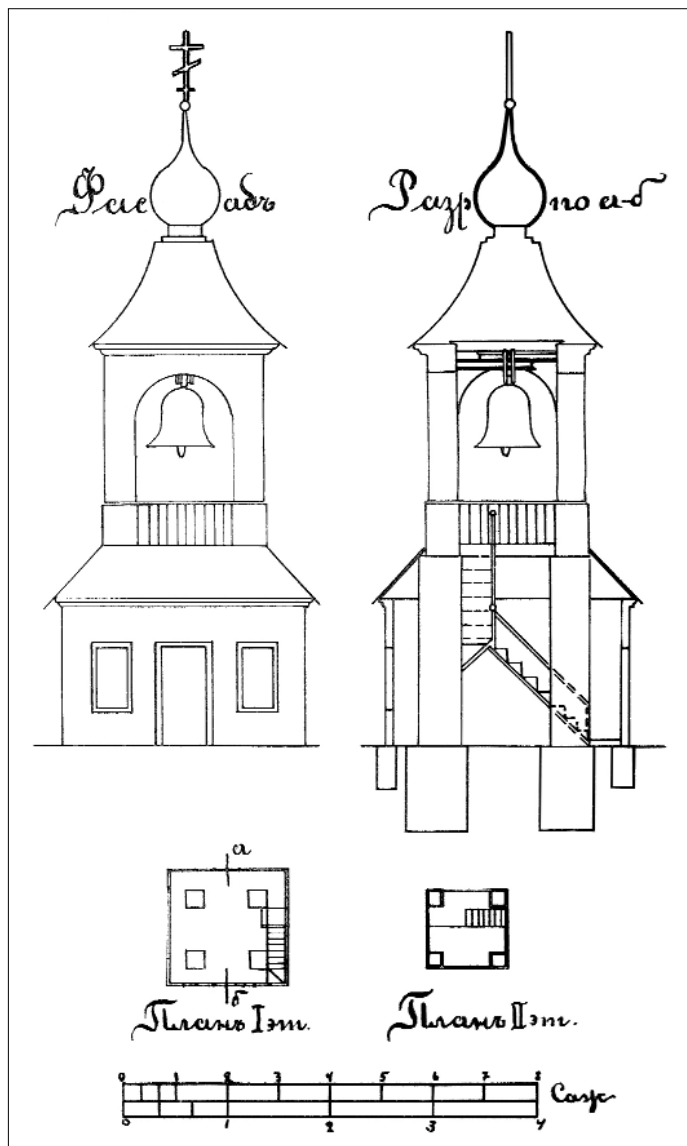
Проект звонницы Преображенского храма в селе Никулино. Из фондов ЦИАМ.
