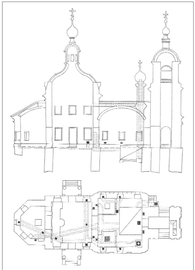
Проект духового отопления церкви в селе Савельево. 1905 год. Из фондов ЦИАМ.
