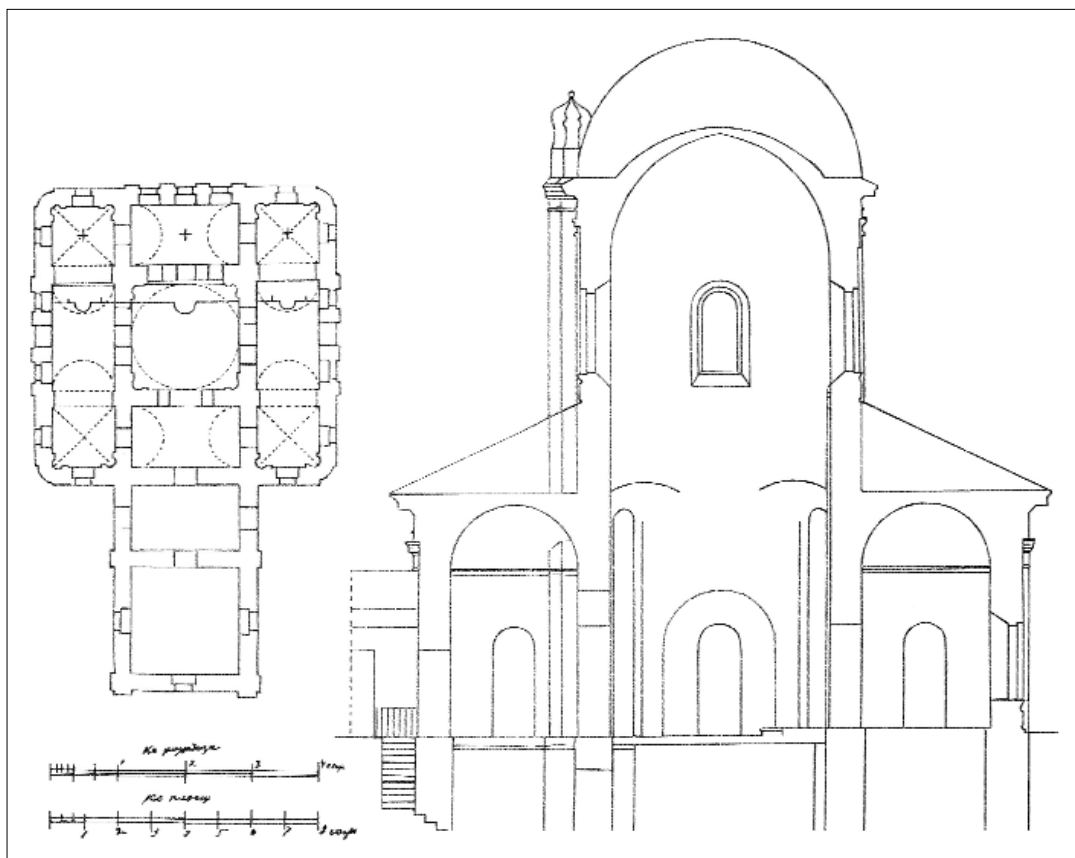
План и разрез Богородицерождественской церкви в селе Надовражино. 1905 год. Из фондов ЦИАМ.
