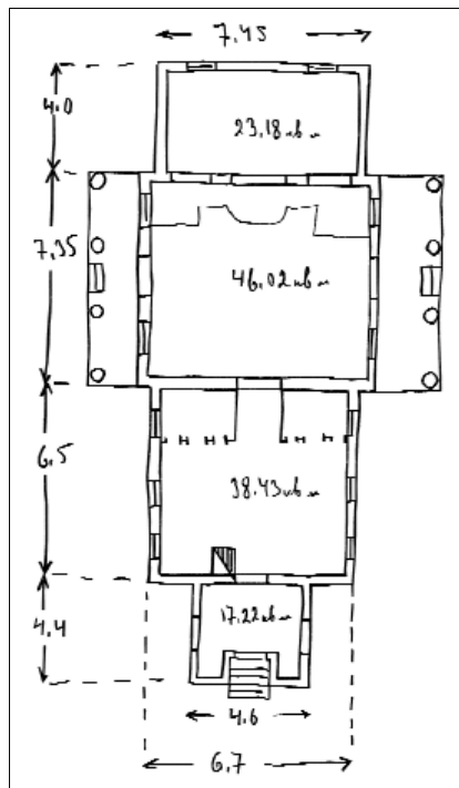
План деревянной Троицкой церкви. 1931 год. Из фондов ЦГАМО.
